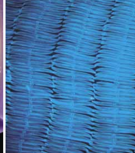
В верхнем ряду слева — детали края створки диатомеи Hyalodiscus . Фото Р. Кроуфорда. В центре и справа — примеры различного преломления света в кремниевом панцире двух видов диатомей (подробнее на с. 55)
