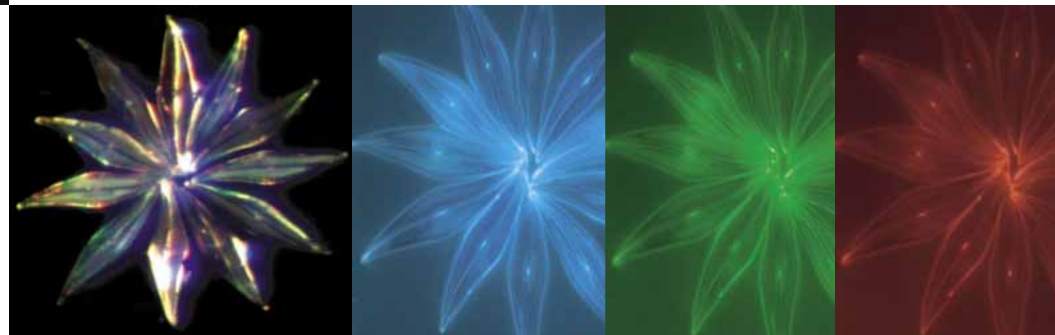
Особое расположение мелких деталей на створках у некоторых видов диатомей может усиливать взаимодействие их «стеклянного» панциря со светом. Первое фото слева — пример преломления света в панцире диатомеи; другие фотографии получены с помощью разных цветных фильтров. Световая микроскопия
