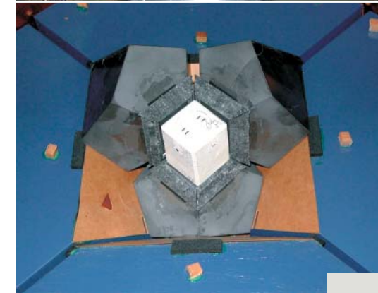
Многоанвонный блок аппарата БАРС (разные стадии сборки)
